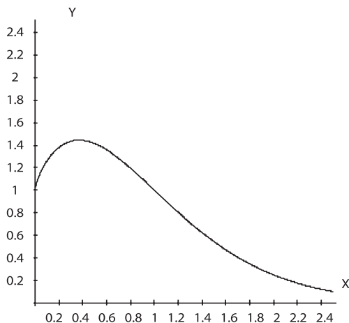
Рис.2. График функции развития y = F(x) = x^{-x} , где x > 0
