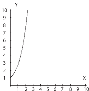
Рис. 1. График зависимости качества от количества P(x) = C e^x , где C = 1
