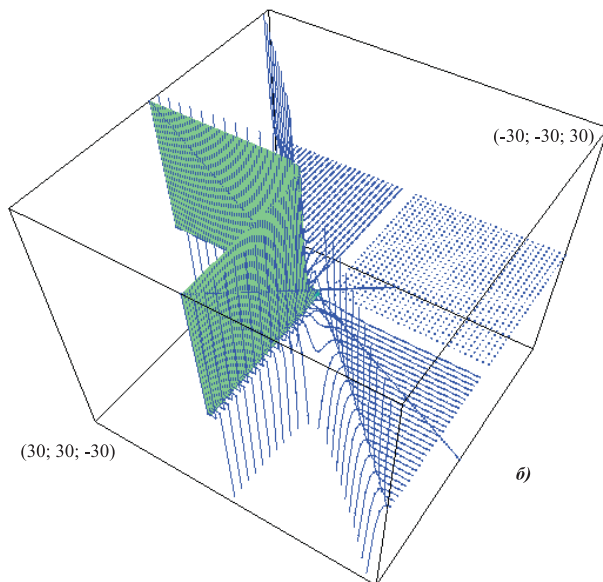
Рис.4. График поверхности функции взаимодействия z = F(x, y) = x^y \cdot y^x
