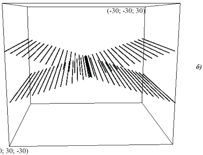
Рис.3. График поверхностей функции взаимодействия z = F(x, y) = x^y \cdot y^x где x + y = 1
