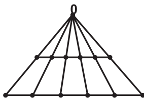
Рис. 5. Соответствие между точками двух отрезков разной длины
